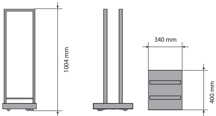
HOLZWAGEN
